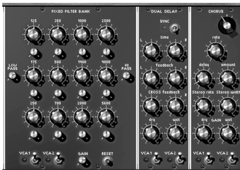
Les 3 modules d'effets
