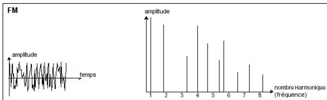
Représentations temporelle et spectrale d'une modulation de fréquence
