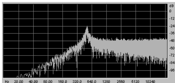
Passe-haut 12 dB/octave
