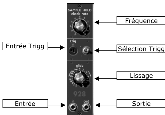
Échantillonneur Bloqueur
