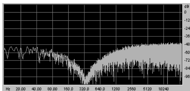
Coupe-bande 24 dB/octave
