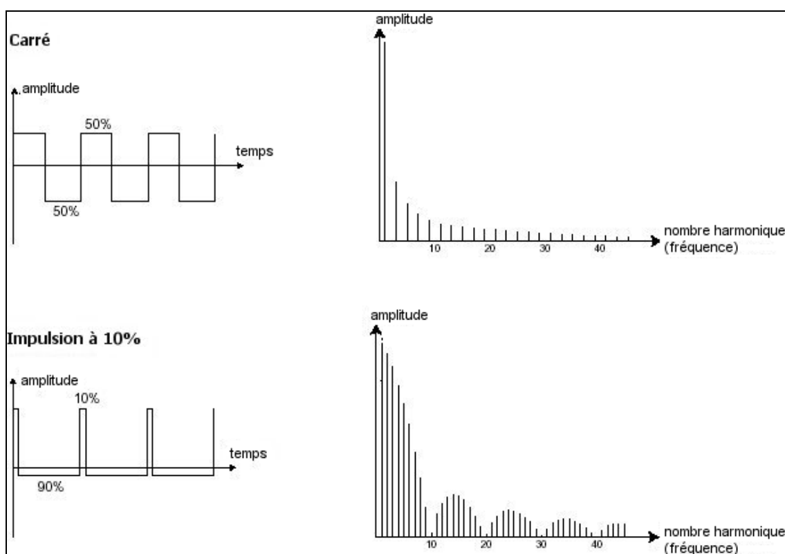
Représentations temporelle et spectrale d'un carré
