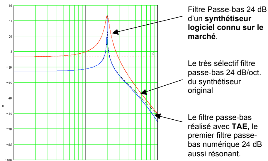
Courbes de réponse des filtres passe bas
