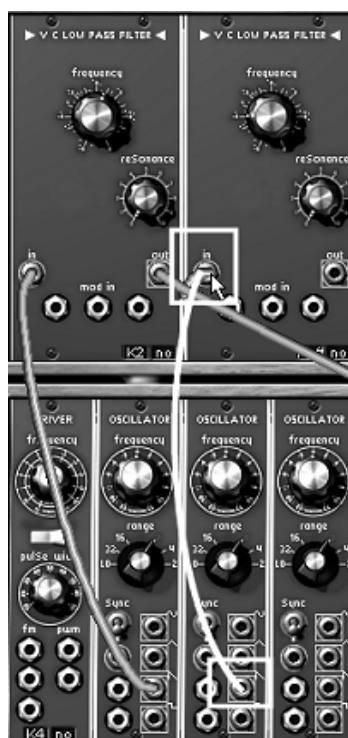
Connexion entre l'oscillateur 2 et le filtre2
