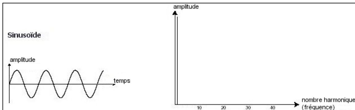
Représentations temporelle et spectrale d'une sinusoïde
