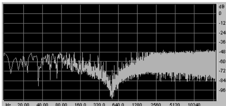
Filtre coupe-bande
