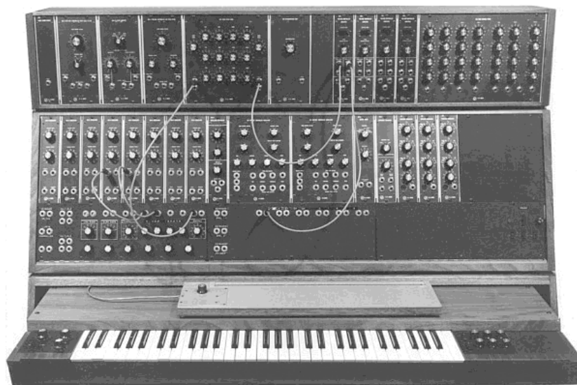
Le système modulaire III (1967)
