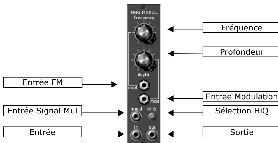
Modulateur en Anneau
