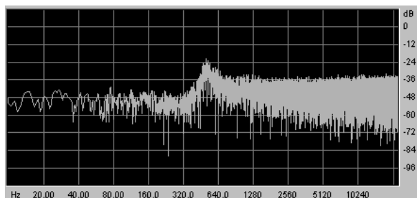
Plateau passe-haut 12 dB/octave
