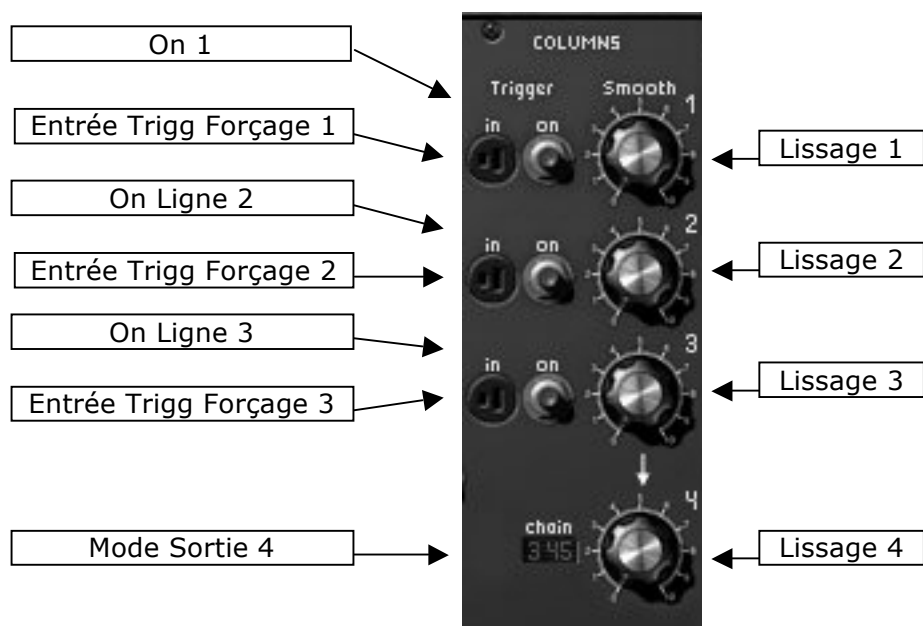
Sorties du séquenceur
