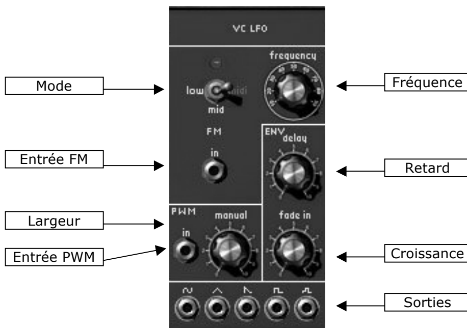
Oscillateur basse-fréquence
