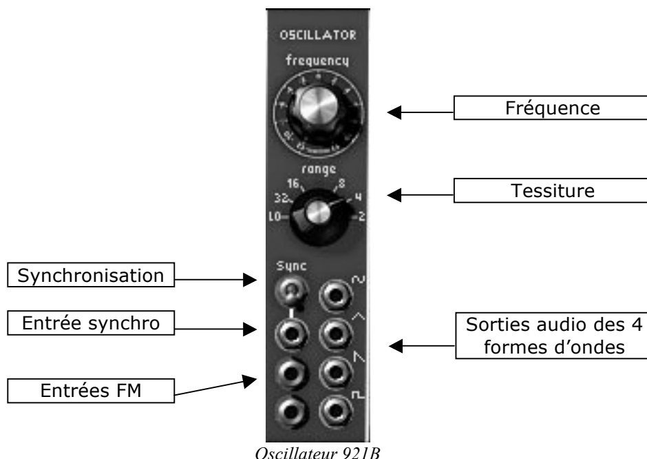
Oscillateur 921B
