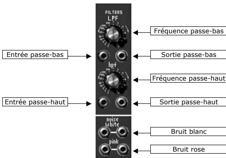
Générateur de bruit
