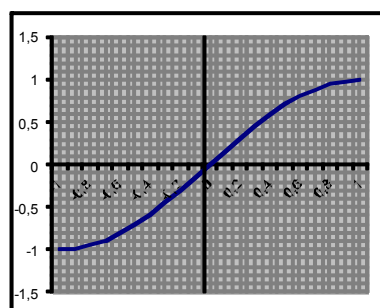
Fonction de transfert du soft clipping
