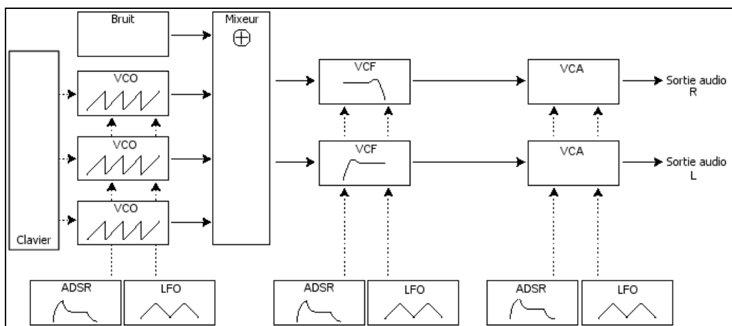
Schéma d'un synthétiseur complet
