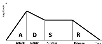
ADSR-Hüllkurven-Abschnitte
